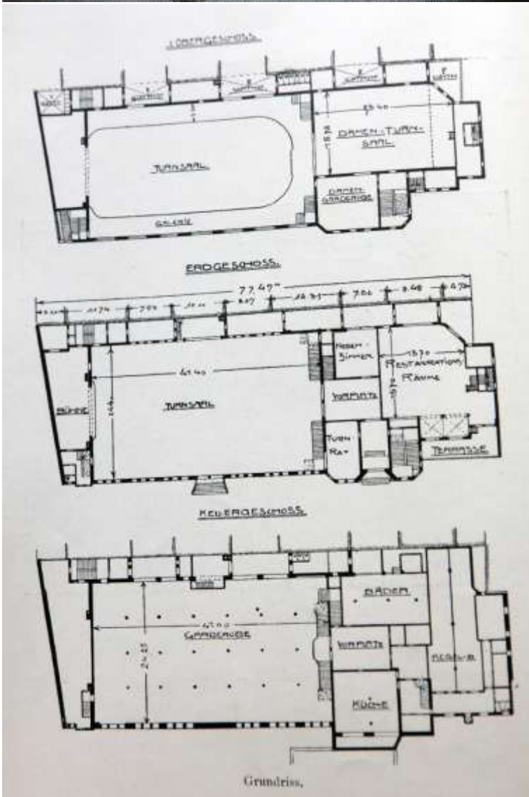
Vereinsgebäude des MTV München um 1909: Halle 1, Halle 2, Baderaum, Kneipe, Grundrisse (Archiv MTV München).
